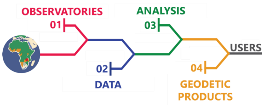
Рисунок 1 Логистическая цепочка в сфере глобальной геодезии.
